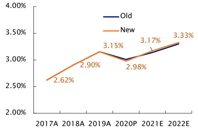
Bảng 4: NIM (%)
